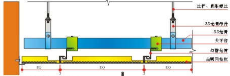
金属网格板安装截面图
