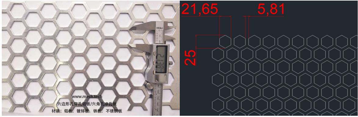
正六边孔冲孔板孔径 21.65*25mm
